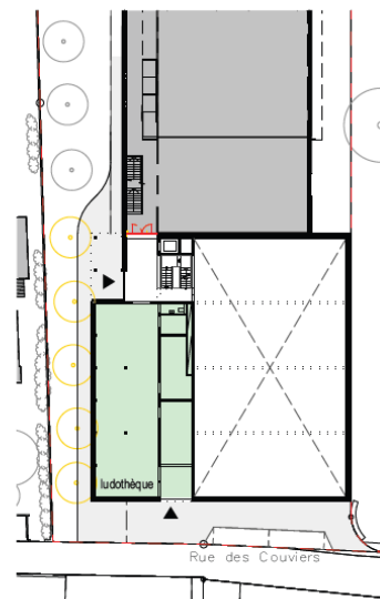
rez-de-chaussée
